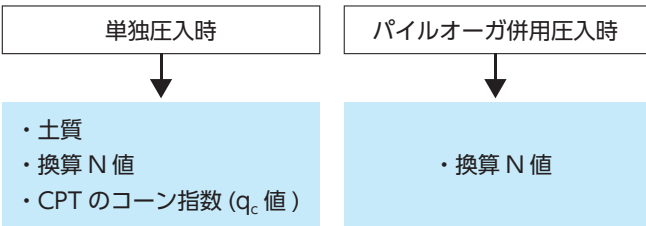
N 値と土質の推定結果
